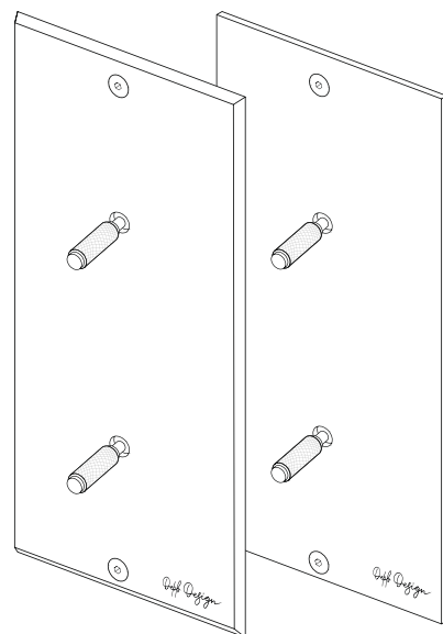
Дизайн пластины с вертикальным расположением винтов
